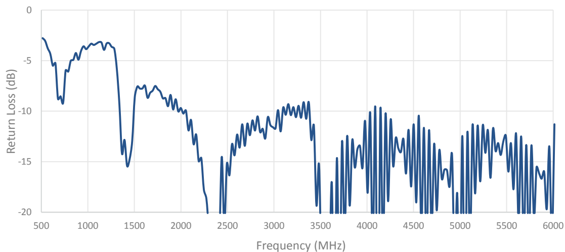
Cable 4: 5GNR
