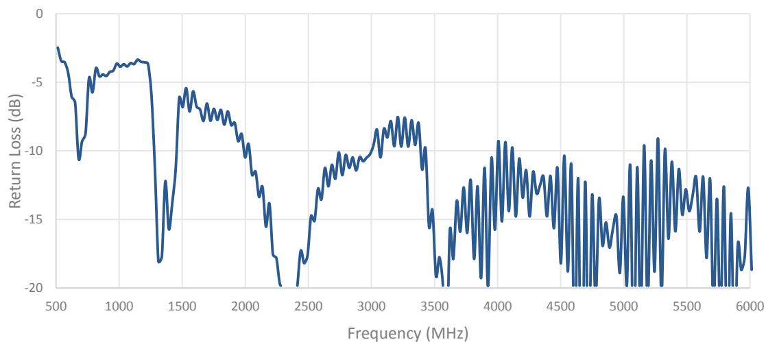
Cable 2: 5GNR
