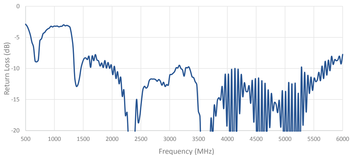
Cable 3: 5GNR
