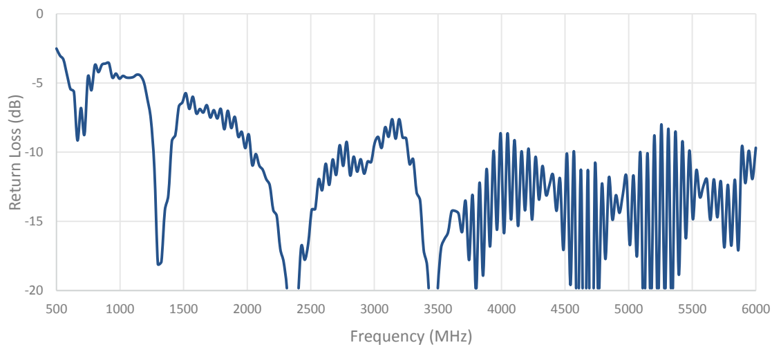
Cable 1: 5GNR
